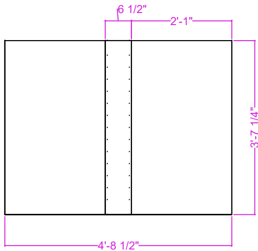
A Elevation
