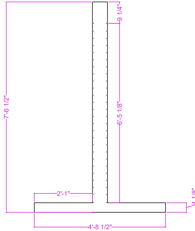
B Elevation
