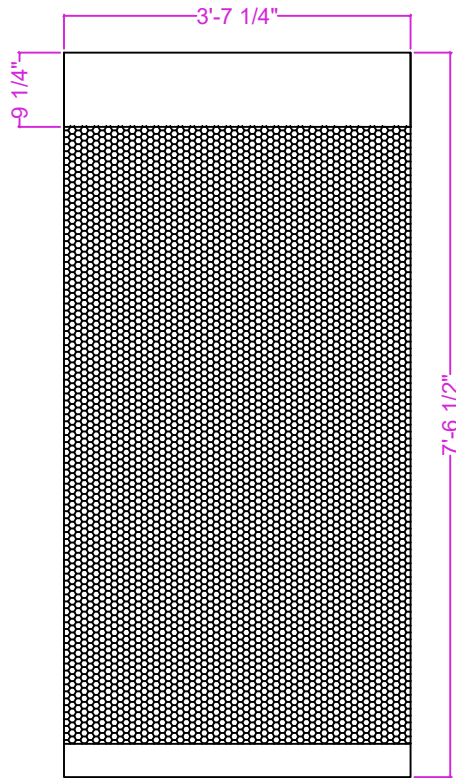
A Elevation
